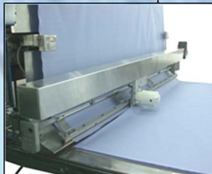
自動數碼定位布長，自動切布 Automatic Digital Fabric Length Positioning and Cutting
