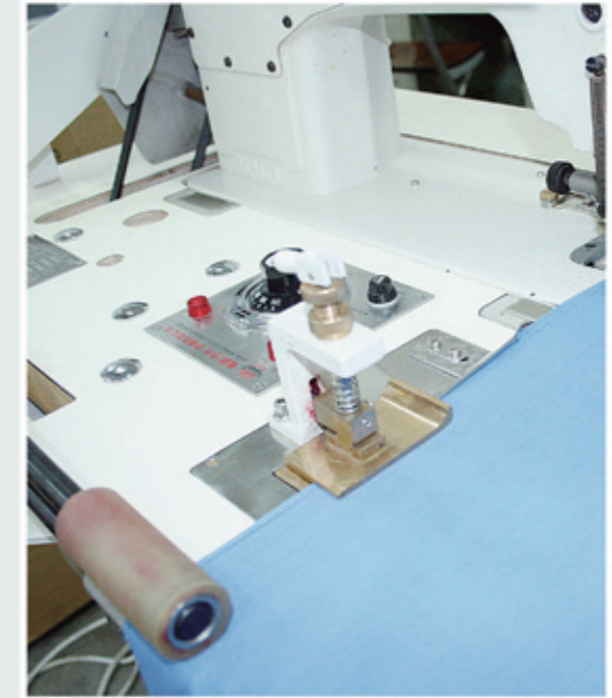
NS-1110 開骨及折紙口 Open seam and fold margin
