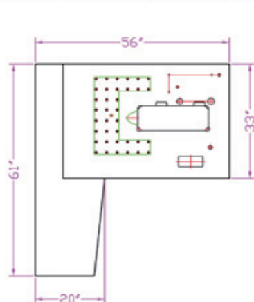
NS-6039-1 工作臺面 Working table size
