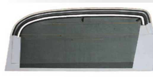
NS-6039-2 男裝西裝內襟夾模 Man's suit lapel stitch jig 最大夾模尺寸：85 x 40cm Max. size of stitch jig: 85 x 40cm
