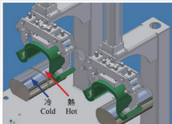
a. 熱壓狀態 Hot creasing status b. 冷壓狀態 Cold creasing status
