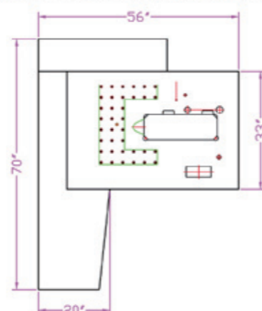
NS-6039-2 工作臺面 Working table size
