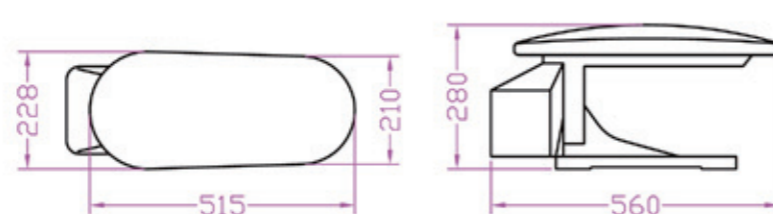
C款尺寸簡圖(標準型) Size of model C(Standard model)
