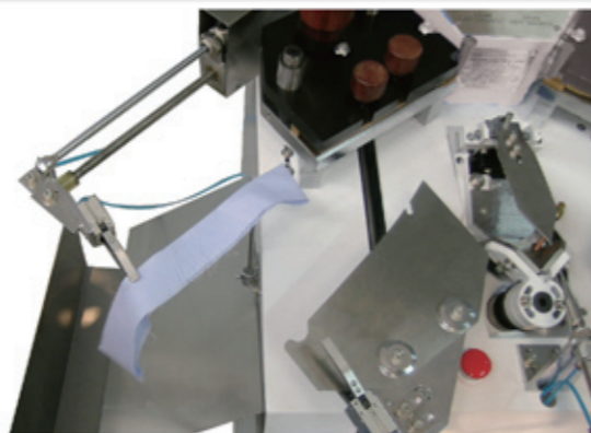
機械手自動收料 Automatic arm for stacking automatically
